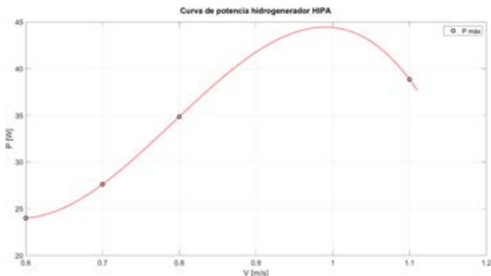
Figura 4. Curva de potencia ( P , expresada en unidades W) generada a diferentes rangos de velocidades
