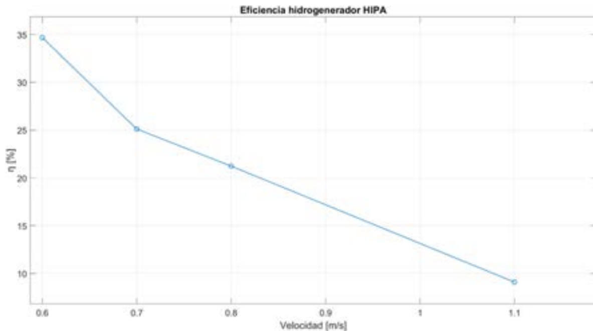
Figura 5 Eficiencia a diferentes velocidades de la corriente
